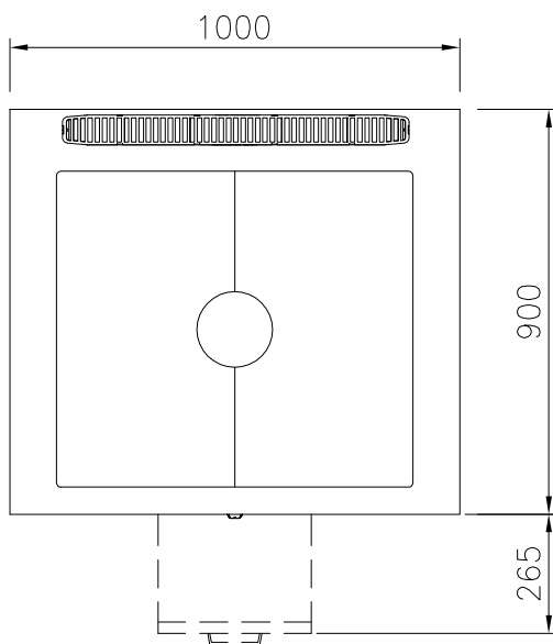
Planta
